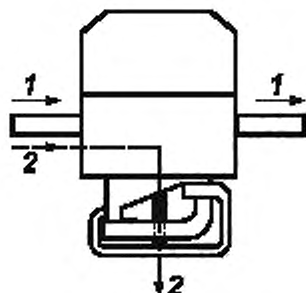
Рисунок 5 — Схема испытания на тепловой кратковременно выдерживаемый ток
