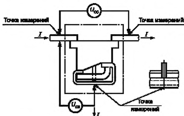
Рисунок 2 — Схема измерений падения напряжения
