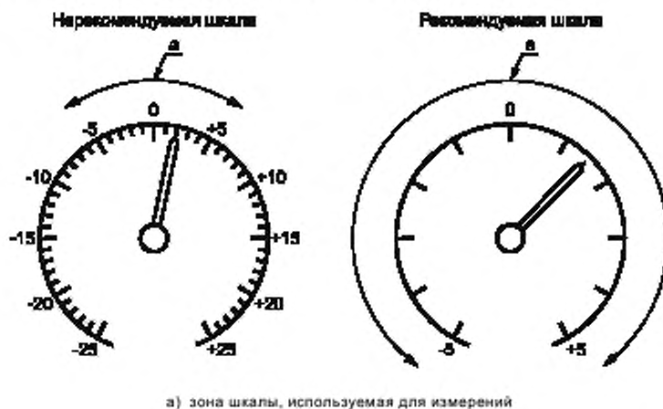
Рисунок 6 — Правильное и некорректное использование шкалы
