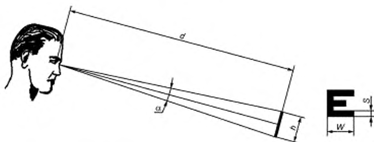
d — дальность наблюдения (расстояние от глаз до знака); \alpha — угловой размер знака; h — высота знака; W — ширина знака; S — толщина штриха в знаке
