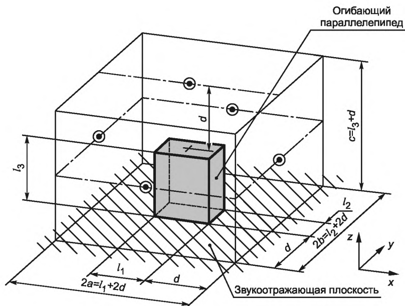
Рисунок В.2 — Пример измерительной поверхности и точки измерения на ней для машин малых размеров [ l_1 \leq d, l_2 \leq d, l_3 \leq 2d ( d — измерительное расстояние, обычно 1 м)]
