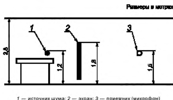
Рисунок А.1 — Схема установки экрана
