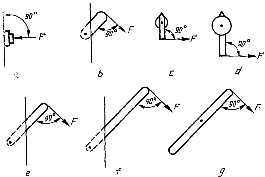
Рисунок 1 — Усилие, прикладываемое к органу управления
