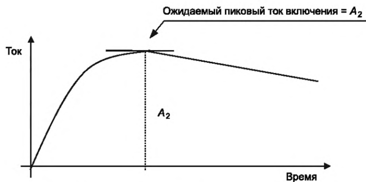
б) Калибровка испытательной цепи на постоянном токе
