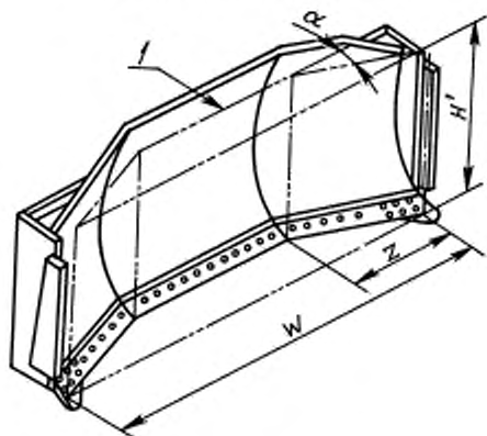
Эффективный контур для сферического и полусферического отвалов
