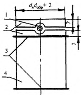
Рисунок 6 — Шарнирное устройство
