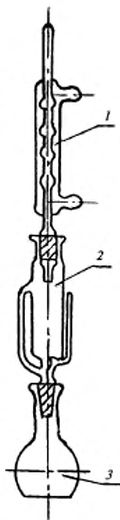
Рисунок 11 — Аппарат типа Соклет
