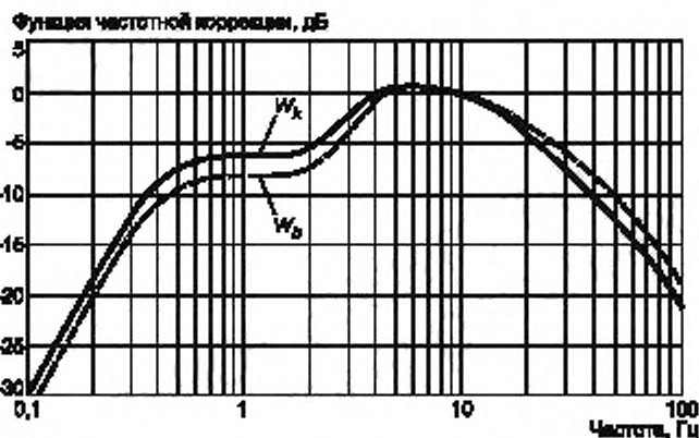
Рисунок 2 — Функции частотной коррекции W_b и W_k
