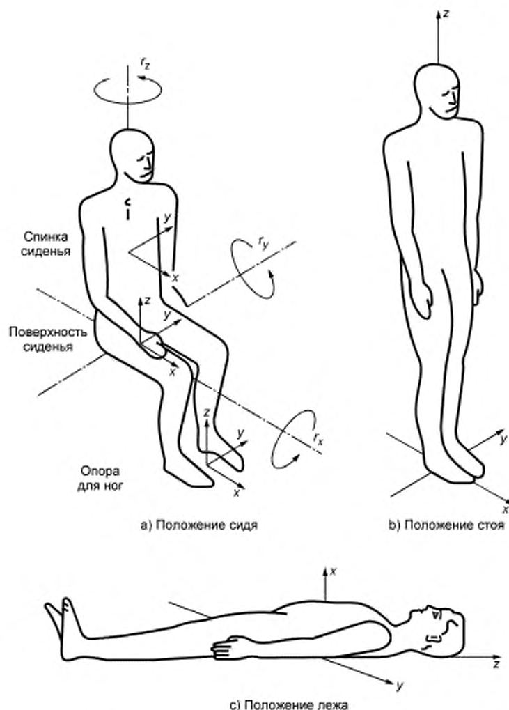
Рисунок 1 — Базицентрическая система координат для тела человека
