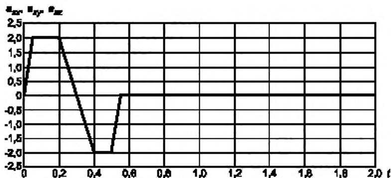
а) Входной сигнал ускорения на подушке сиденья
