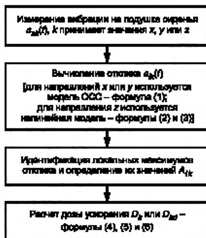
Рисунок 1 — Блок-схема расчета дозы ускорения
