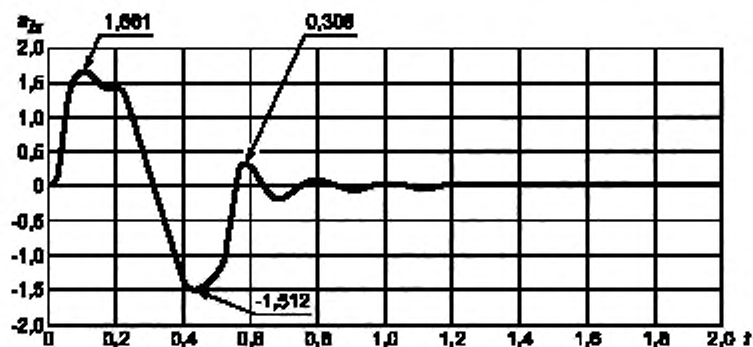
c) Реакция позвоночника в направлении z
