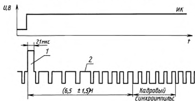
Структура испытательного сигнала И
