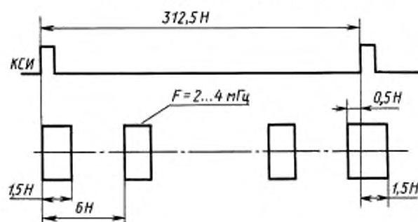
Структура испытательного сигнала И
