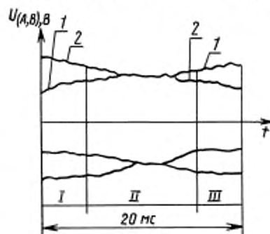
Предварительное выставление параметра X
