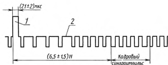
1 — маркер; 2 — уровень черного
