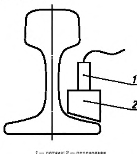
Рисунок 2 — Точка измерения на подошве рельса
