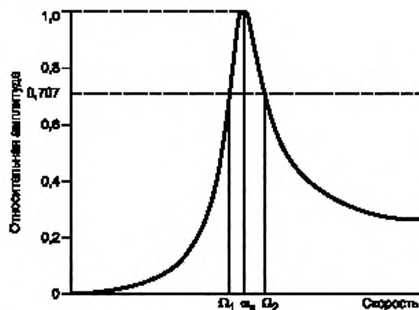
Рисунок 5 — Диаграмма Бode для оценки модальной чувствительности
