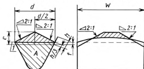
Ковш с непрямолинейной режущей кромкой
