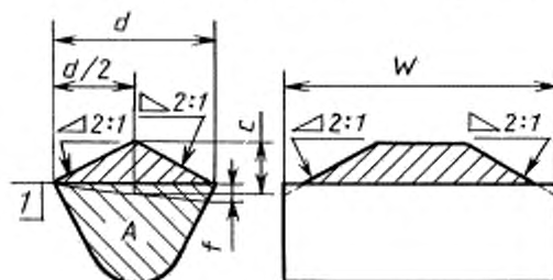
Ковш с выступающей прямолинейной кромкой
