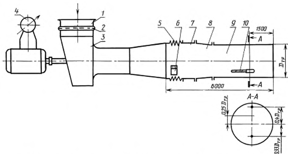
1 — коллектор; 2 — дросселирующее устройство; 3 — ТДМ; 4 — ваттметр; 5 — гибкая вставка; 6 — ОИШ; 7 — промежуточный участок; 8 — переходный участок; 9 — измерительный участок; 10 — измерительный микрофон с ветрозащитной насадкой
