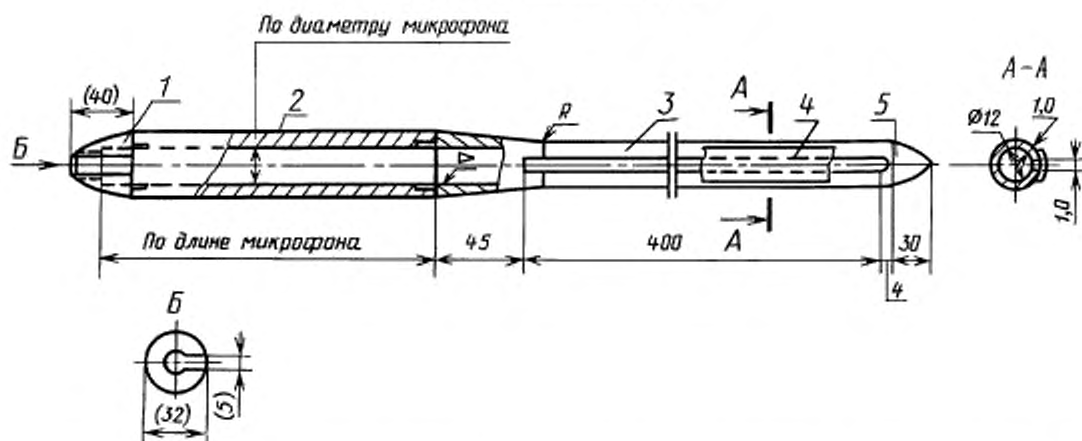
Насадка на дюймовый микрофон
