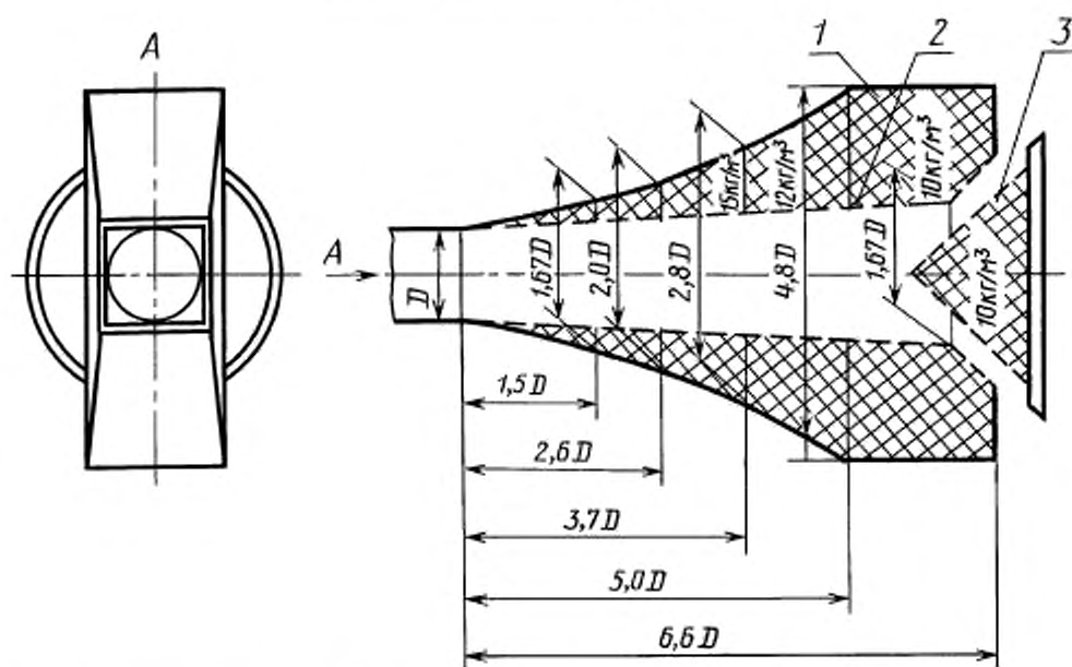
Схема концевой поглощающей устройства
