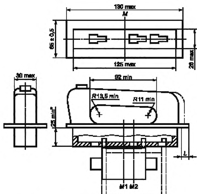
Рисунок 3 (I) — Съёмная ручка для смены плавкой вставки
