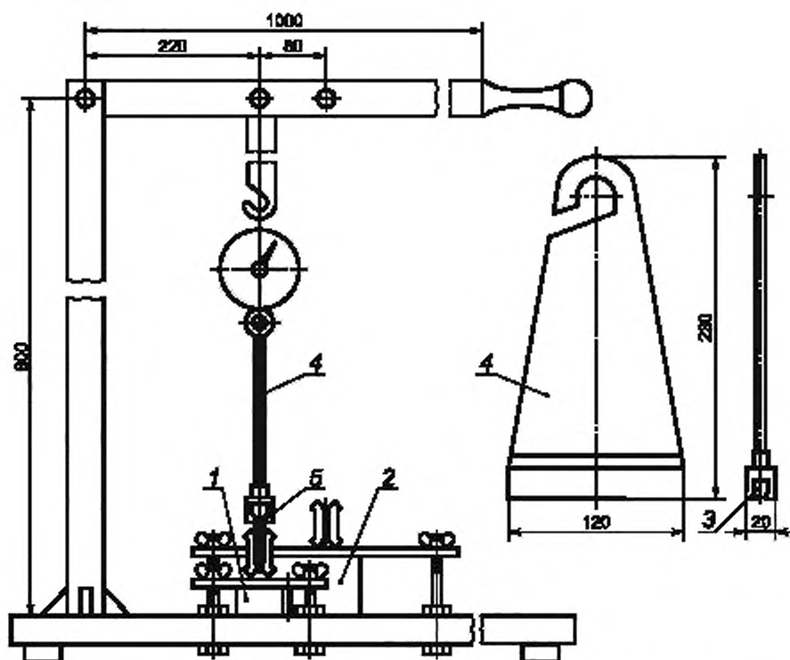
1 — основание плавкого предохранителя габарита 00; 2 — основание плавких предохранителей других габаритов; 3 — размеры, достаточные для монтажа креплений плавкой вставки; 4 — металлический лист; 5 — испытательный нож
