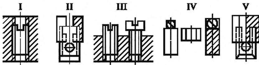
Рисунок 0 (III) — Виды зажимов
