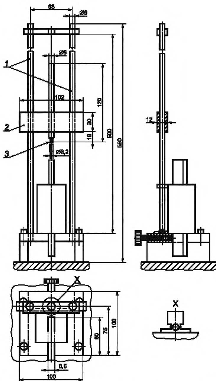
1 — направляющие; 2 — молоток (стальной, массой 300 г, высота падения 300 мм); 3 — ударник
