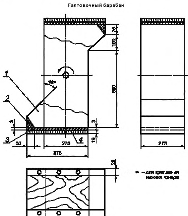
1 — лист из слоистого пластика; 2 — резина; 3 — сталь; 4 — деревянный блок
