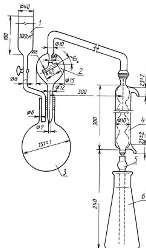
1 — цилиндрическая загрузочная воронка с крапом; 2 — предохранительный объем; 3 — круглодонная колба; 4 — холодильник; 5 — расширительный резервуар; 6 — приемная колба
