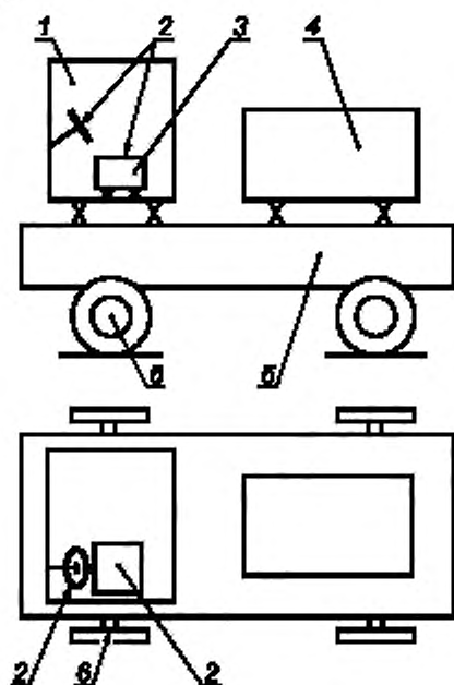
1 — кабина; 2 — точка измерения параметра вибрационной характеристики (сиденье, рулевое колесо); 3 — сиденье; 4 — двигатель; 5 — рама; 6 — контрольная точка (ступица колеса)
