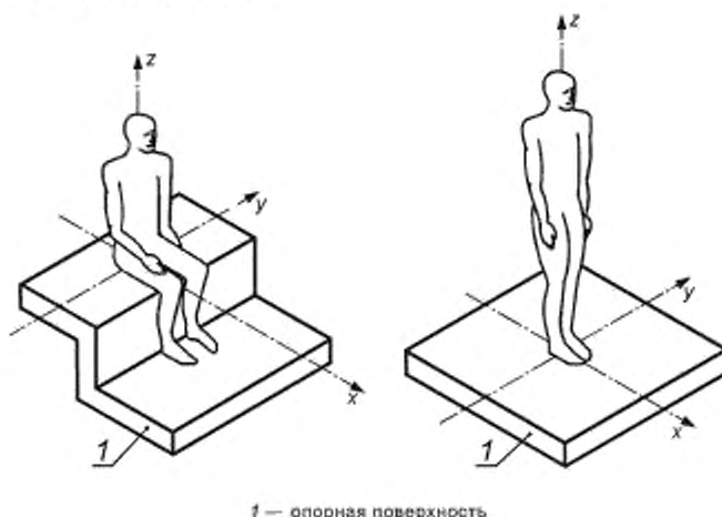
Рисунок 1 — Направления осей базисной системы координат
