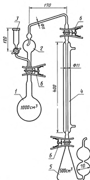
Дистилляционный аппарат
