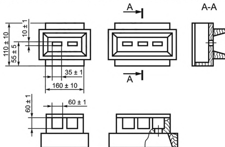
Рисунок А.1 — Компаратор
