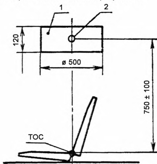
1 – прозрачный цилиндр; 2 – центр цилиндра
