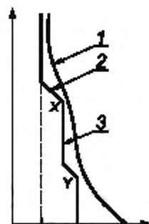
1 — преддугловая характеристика; 2 — прямая постоянного значения I^2t ; 3 — условная кривая перегрузок
