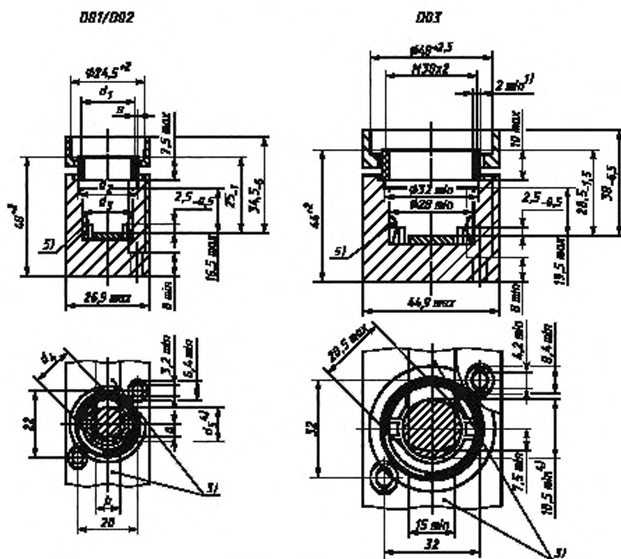
Рисунок 1 — Основные размеры плавких вставок предохранителей типа D
