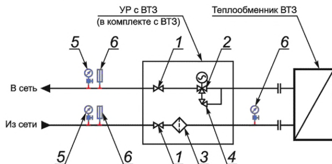
Узел регулирования воздушно-тепловой завесы автостоянки
