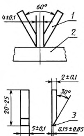
1 — электрод; 2 — образец; 3 — слеска закрученный край
