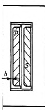
Двойной и более каркас
