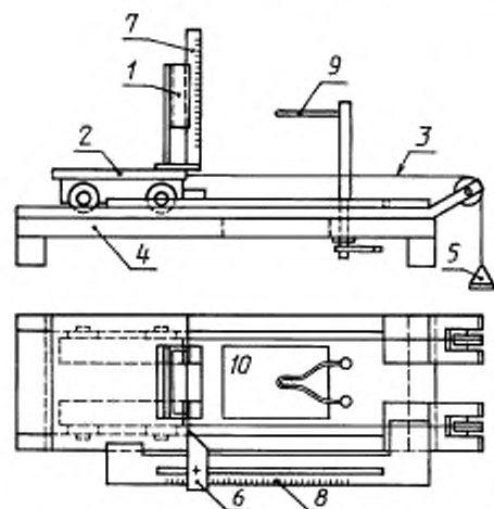
1 — регулирующий зажим положения; 2 — тележка; 3 — натяжной шнур; 4 — опорная плита; 5 — пруж; 6 — регулируемый упор; 7 — масштабная линейка для измерения высоты пламени; 8 — масштабная линейка для измерения глубины проникновения проволоки накала; 9 — проволока накала (рисунок 6); 10 — отверстие в опорной плите
