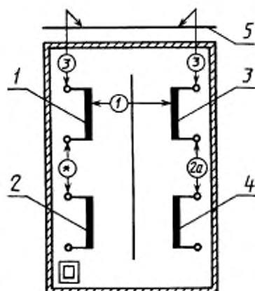
1 — первичная 1; 2 — первичная 2; 3 — вторичная 1; 4 — вторичная 2; 5 — металлическая фольга
