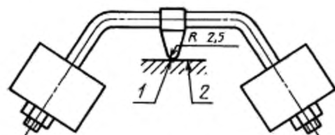
1 — сферическая часть; 2 — образец
