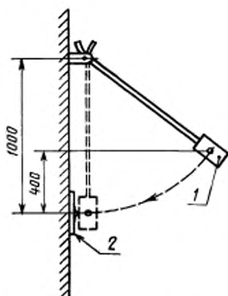
1 — образец; 2 — стальной опорный прямоугольник
