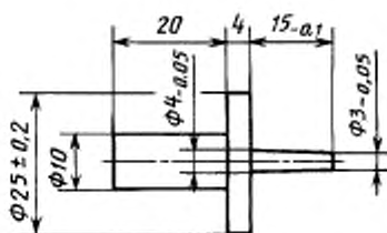
Рисунок 4 — Испытательный стержень
