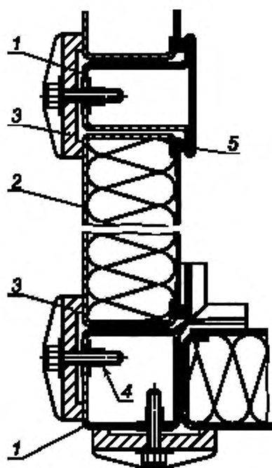
1 — каркас; 2 — стенка; 3 — зажим; 4 — закладная гайка; 5 — резиновое уплотнение
