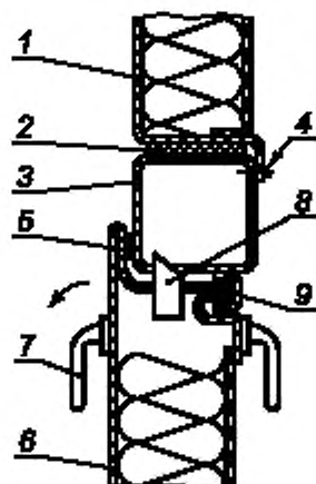
1 — стенка; 2 — самоклеящееся резиновое уплотнение; 3 — рама двери; 4 — винтовое соединение; 5 — первое дверное уплотнение; 6 — дверь; 7 — дверная ручка; 8 — запор замка; 9 — второе дверное уплотнение
