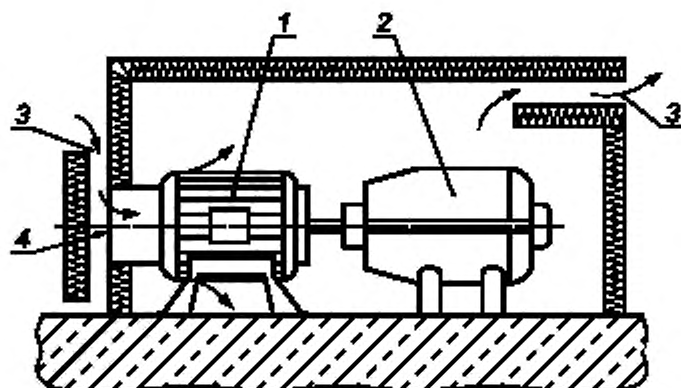
1 — электромотор; 2 — турбокомпрессор; 3 — акустически защищенные всасывающий и выпускной воздуховоды; 4 — защитная сетка
