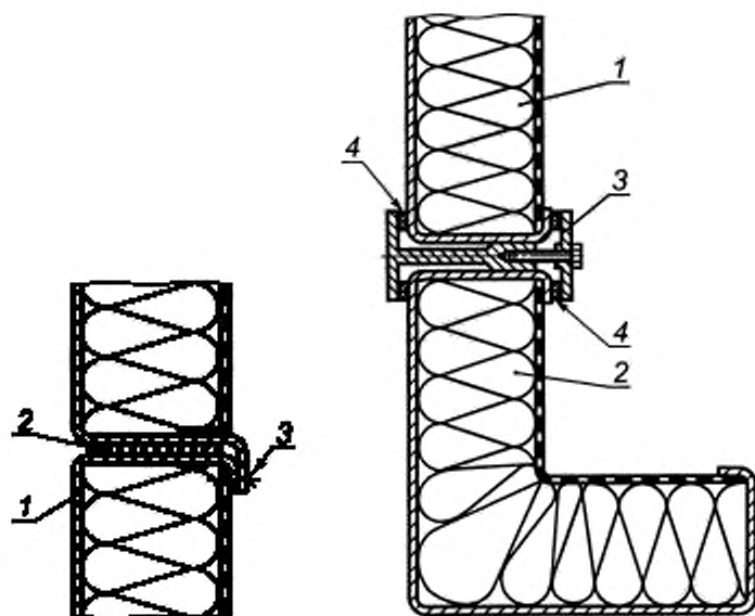
1 — стенка; 2 — самоклеящееся резиновое уплотнение; 3 — винтовое соединение
