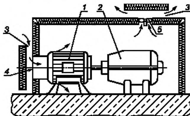
1 — электромотор; 2 — турбокомпрессор; 3 — акустически защищенные всасывающий и выпускной воздуховоды; 4 — защитная сетка; 5 — вентилятор
