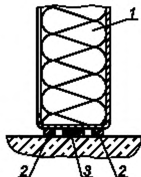
1 — стенка; 2 — жесткий стальной профиль; 3 — резиновый уплотнитель
