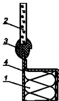
1 — стенка; 2 — оконное стекло толщиной не менее 6 мм; 3 — резиновое уплотнение; 4 — кромка оконного проема
