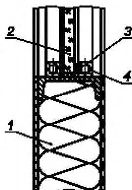
1 — стенка; 2 — оконное стекло толщиной не менее 6 мм; 3 — резиновое уплотнение; 4 — монтажный профиль
