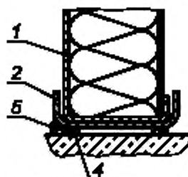
б) На неровном (бетонном) полу
