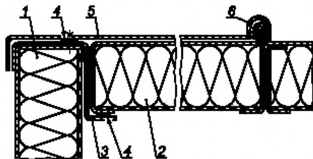
1 — стенка; 2 — потолочная панель; 3 — несущий профиль; 4 — резиновое уплотнение; 5 — защищающая от осадков кровля; 6 — защищающий от осадков кожух
