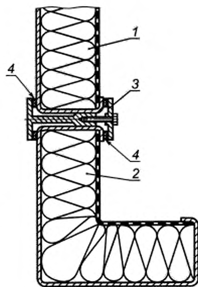
1 — стенка; 2 — угловой элемент; 3 — соединительный элемент с устройством регулировки (длинные профили); 4 — резиновое уплотнение
