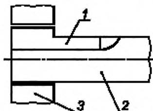
1 — шпонка в виде ступеньки; 2 — вал; 3 — насадка
