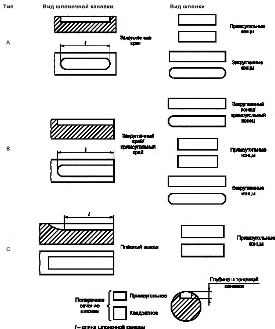
Рисунок 1 — Основные виды шпонок и шпоночных канавок
