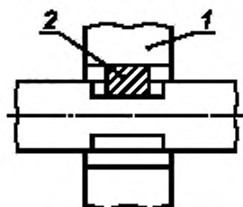
1 — насадка; 2 — шпонка половинной длины
