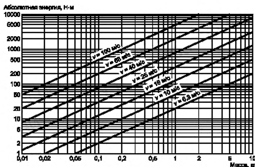
Рисунок А.4 — Зависимость абсолютной энергии от массы и поступательной скорости частицы
