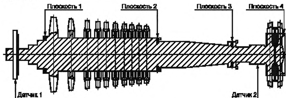
Рисунок D.1 — Ротор турбины
