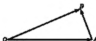
Рисунок G.1 — Векторный эффект установки пробных масс
