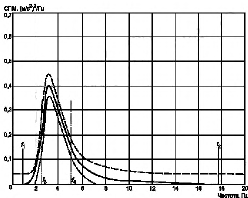
Рисунок 3 — СПМ для спектрального класса IT 2 (категория 4a)
