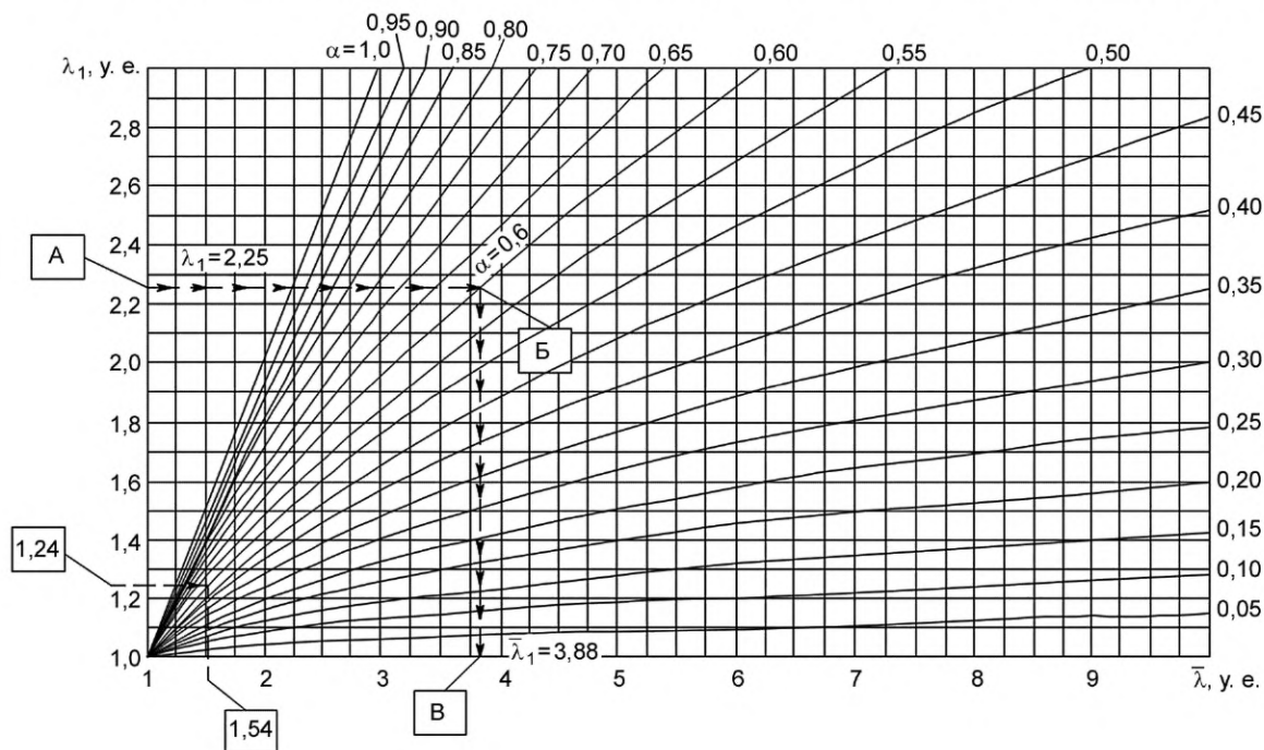
Рисунок A.4 — Номограмма к примеру определения значения показателя среднего размера \bar{\lambda} открытых капиллярных пор (при вспомогательном параметре \lambda_1 \geq 1 )
