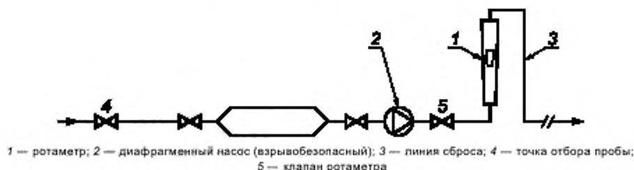
Рисунок С.3 — Отбор проб в стеклянные пипетки при давлении в газопроводе ниже атмосферного
