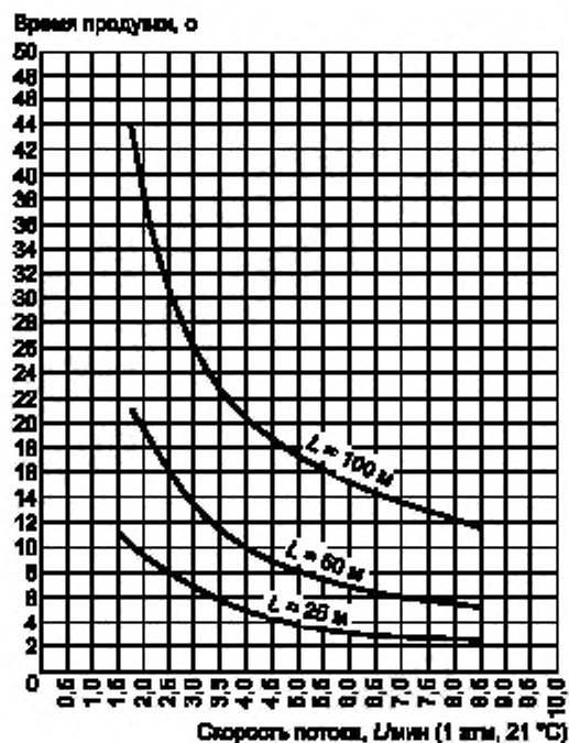
Рисунок G.5 — Время продувки как функция скорости потока (внутренний диаметр трубки — 4 мм)
