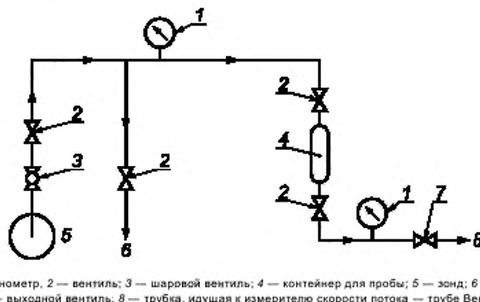
Рисунок Е.1 — Схема отбора проб методом контролируемой скорости
