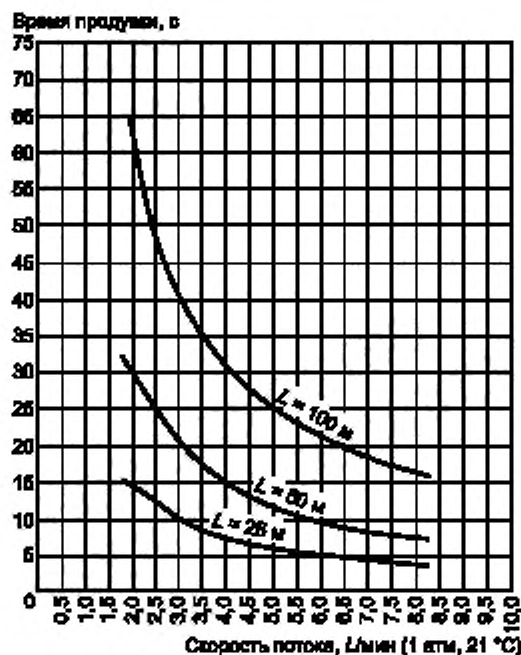
Рисунок G.6 — Время продувки как функция скорости потока (внутренний диаметр трубки — 5 мм)
