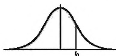
Рисунок Н.1 — Процентильные значения t_p для t-распределения Стьюдента с \nu степенями свободы (заштрихованная площадь = p )
