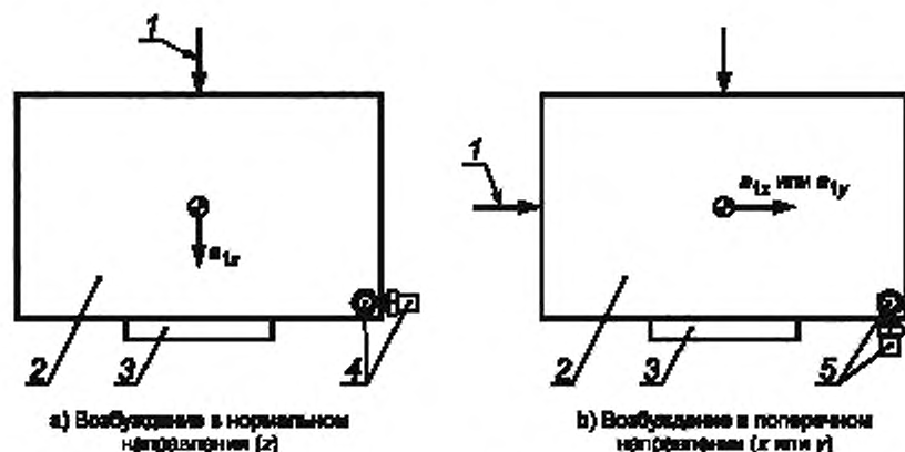
1 — вибровозбудитель; 2 — масса распределения возбуждения; 3 — входной фланец испытуемого объекта; 4 — датчик измерения нежелательной вибрации a'_{1x} и a'_{1y} ; 5 — датчик измерения нежелательной вибрации a'_{1z} и a'_{1y} или a'_{1x}
