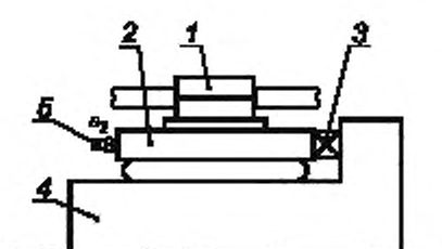
с) Измерение силы на выходной стороне с применением направляющей системы
