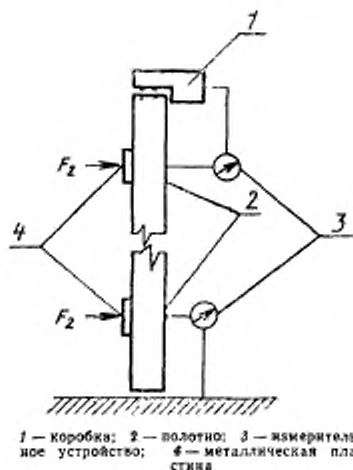
Рисунок 4 — Схема измерения перемещений под нагрузкой F_2
