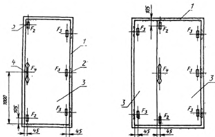
1 — коробка; 2 — петли; 3 — полотно; 4 — закрывающий прибор; 5 — металлическая пластина
