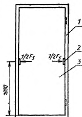
1 — коробка; 2 — металлическая пластина; 3 — полотно
