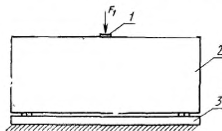
1 — засов замка; 2 — полотно; 3 — жесткая опора
