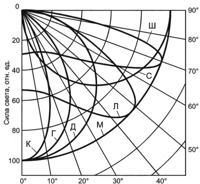
Рисунок В.1 — Типовые меридиональные КСС светильников
