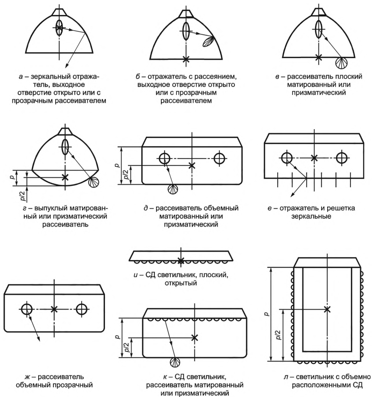
Рисунок А.1 — Положение фотометрического центра осветительных приборов по [2]
