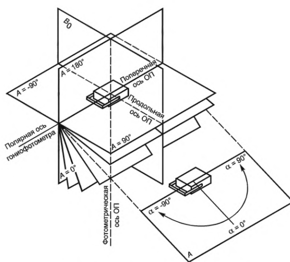
в — система фотометрирования A- \alpha
