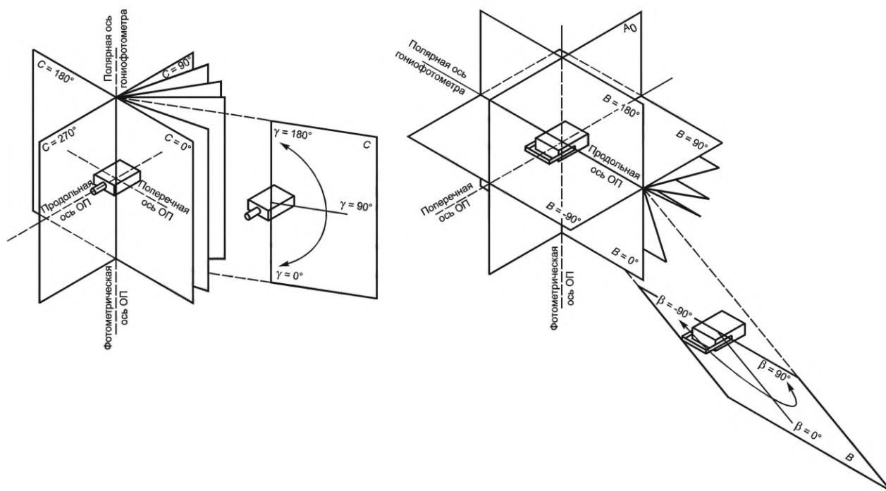
а — система фотометрирования C- \gamma
