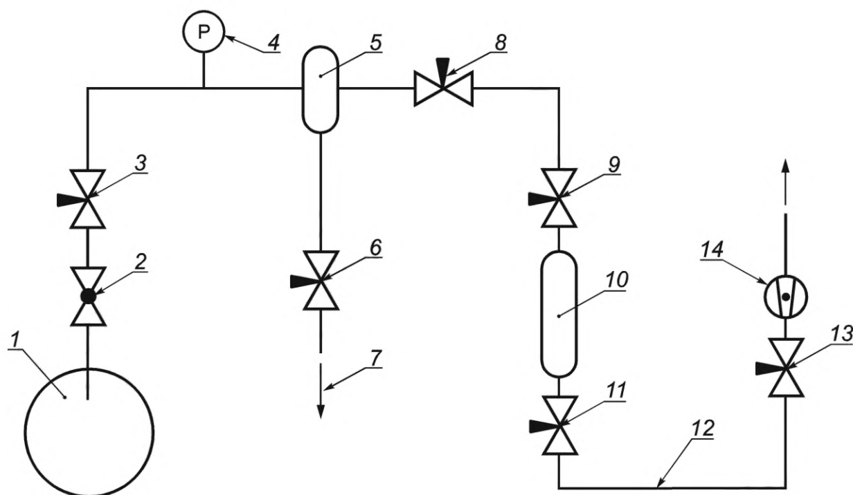
1 — точка отбора проб; 2 — шаровой кран; 3, 8, 13 — вентили; 4 — манометр; 5 — каплеуловитель; 6 — продувочный вентиль; 7 — сброс газа; 9, 11 — входной и выходной вентили пробоотборного контейнера; 10 — пробоотборный контейнер; 12 — отводная линия; 14 — СИ расхода
