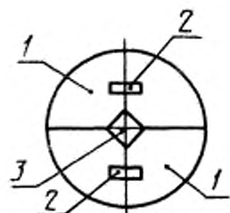
1 — полуфидер; 2 — подшпильное отверстие; 3 — отверстие для инокулята
