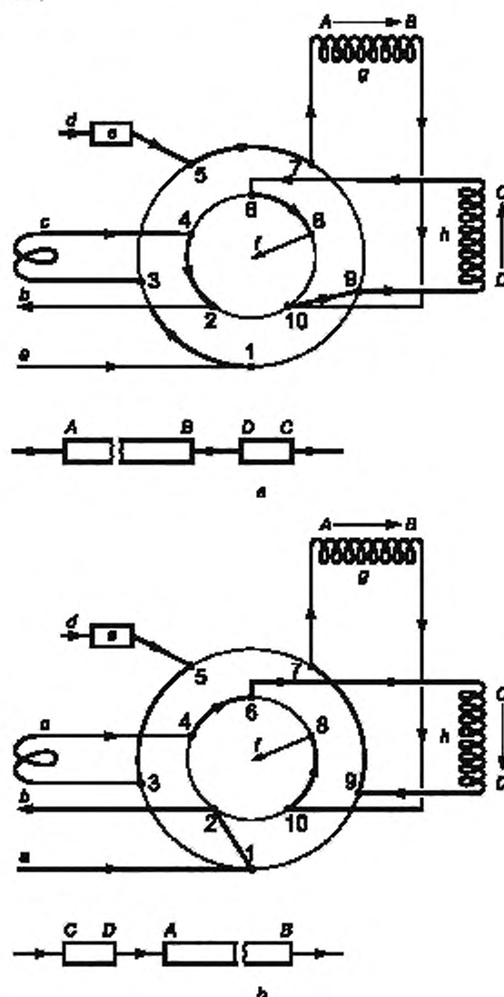
а — проба газа, б — сброс; с — петля крана-дозатора объемом 1 мл; d — газ-носитель; e — ДТП (сравнительный канал); f — ДТП (канал анализа); g — колонка 2 (длина 9 м); h — колонка 2 (длина 0,45 м)
