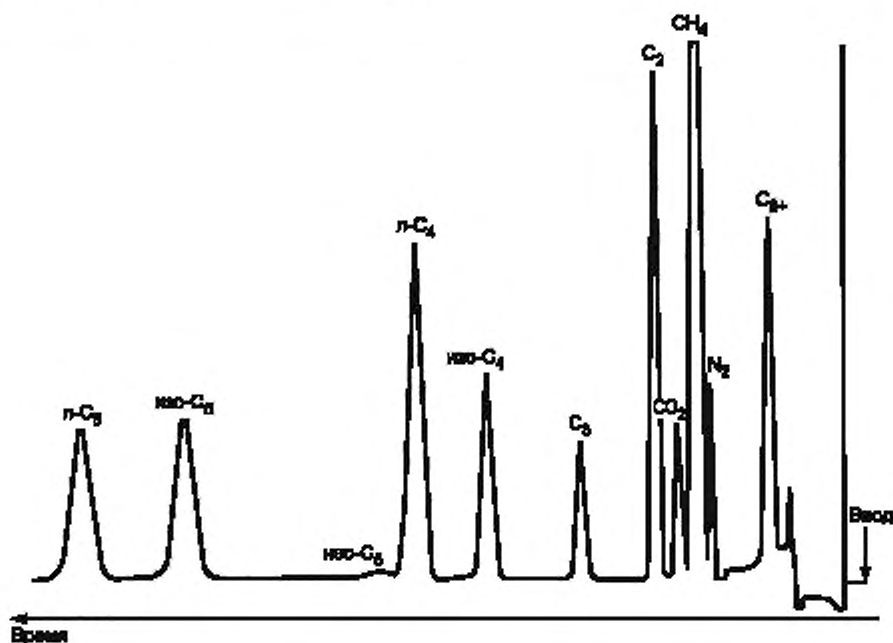
Рисунок 2 — Пример типичной хроматограммы
