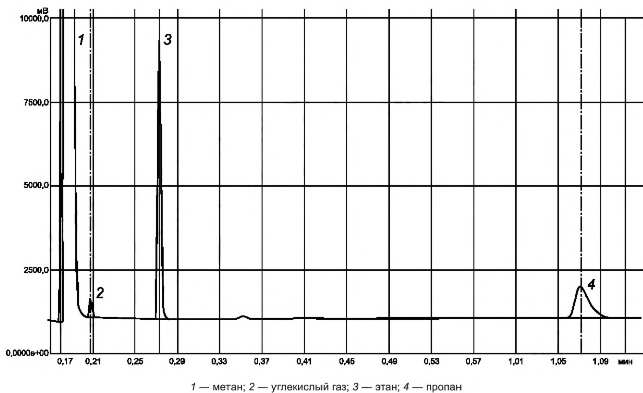
Рисунок Д.1 — Хроматограмма, полученная на канале 1
