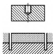
Рисунок 9 — Разрушение по слою клея (испытание следует повторить)
