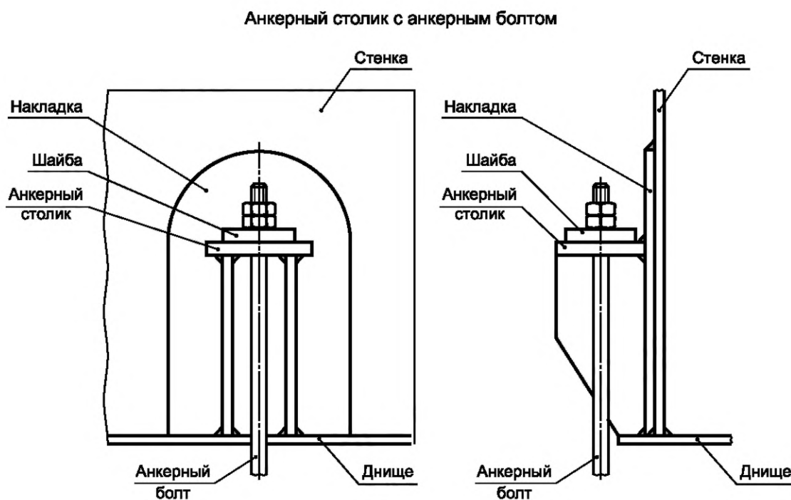
Рисунок 20, лист 1 — Крепление стенки анкерными болтами
