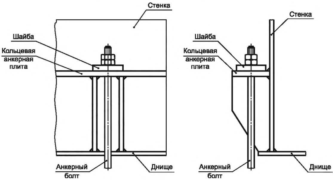
Кольцевая анкерная плита с анкерными болтами
