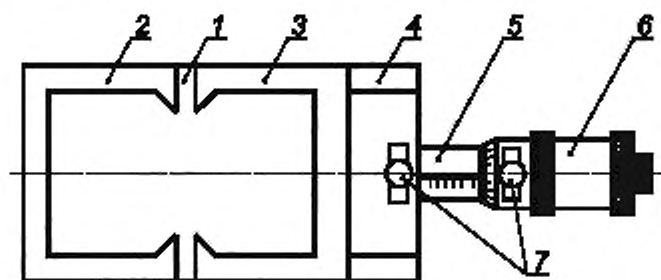
1 — основание; 2 — упорная планка; 3 — подвижный П-образный захват; 4 — неподвижный захват; 5 — внутренний цилиндр растягивающего механизма; 6 — наружный цилиндр растягивающего механизма; 7 — зажимные винты
