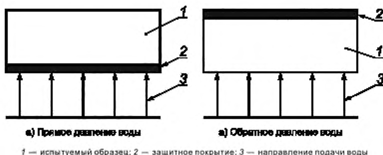
Рисунок 10 — Схема испытаний образцов бетона с покрытием
