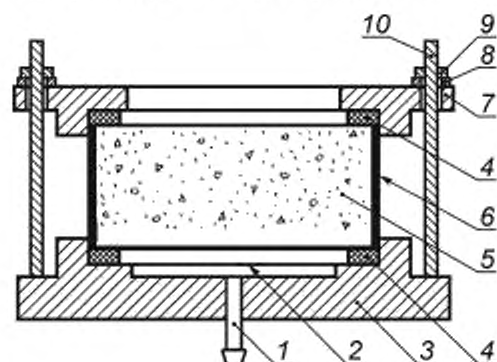
1 — штуцер для подачи воды; 2 — защитное покрытие; 3 — неподвижное гнездо для установки образца; 4 — уплотнительные резиновые кольца; 5 — испытуемый образец; 6 — герметизирующая обмотка или прокладка; 7 — съемная верхняя обойма; 8 — шайба; 9 — гайка; 10 — анкерный стержень с резьбой
