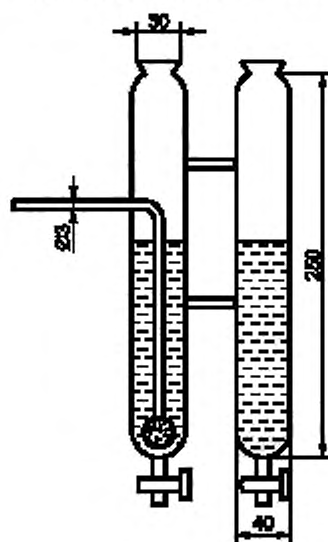
Рисунок 2 — Поглотительный сосуд
