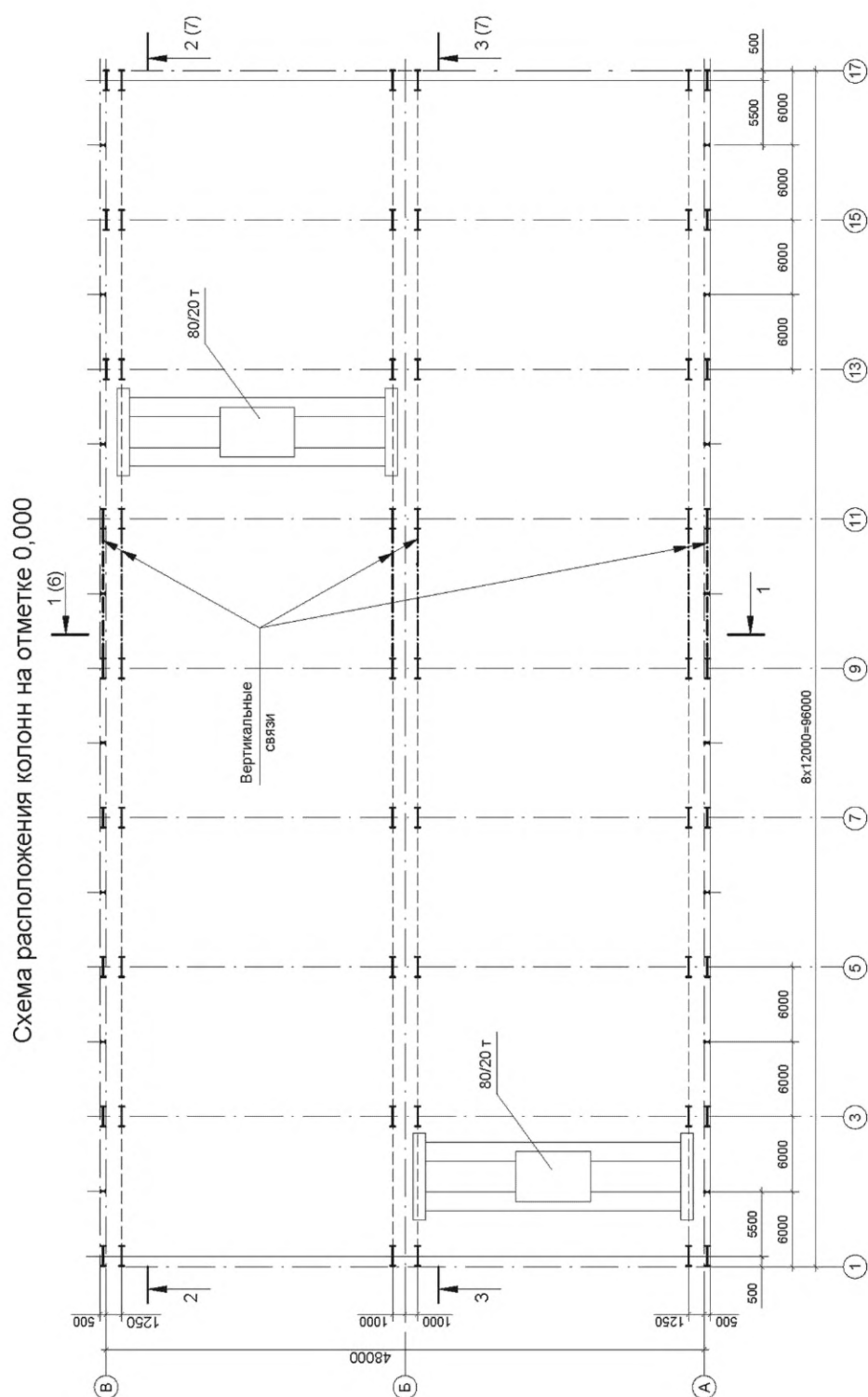
Рисунок Г.3 — Пример выполнения колонн производственного здания
