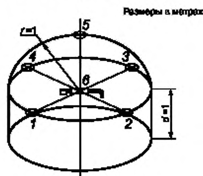
1 — 5 — точки измерений; б — геометрический центр ручной машины; r — измерительный радиус
