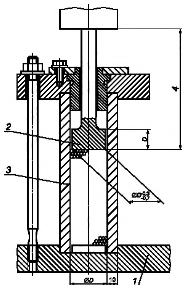
1 — стальная плита основания; 2 — поршень вставного инструмента [сталь твердостью (55 \pm 2) HRC]; 3 — гильза поглотителя энергии [сталь твердостью (62 \pm 2) HRC]; 4 — вылет вставного инструмента
