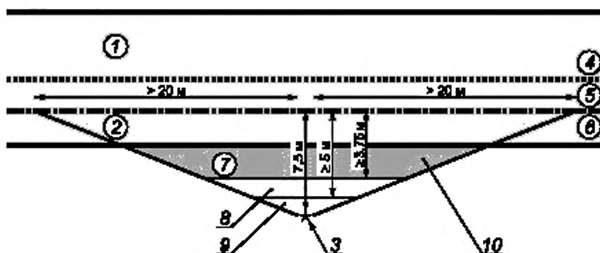
б) Минимальная зона покрытия с заданными акустическими характеристиками между испытуемой полосой дороги и микрофоном
