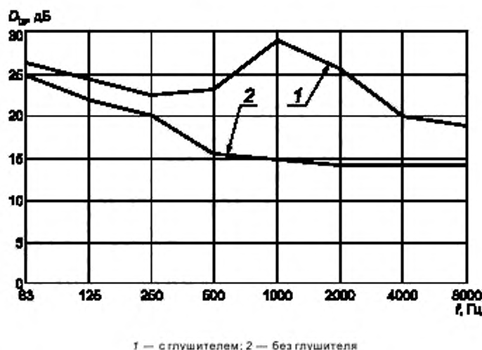
Рисунок А.2 — Зависимость потерь при прохождении D_{15} от частоты f для перекрестного глушителя (гибкий трубчатый глушитель длиной 500 мм, толщина звукопоглощающего покрытия 25 мм) с дисковым клапаном номинальной ширины 150 мм
