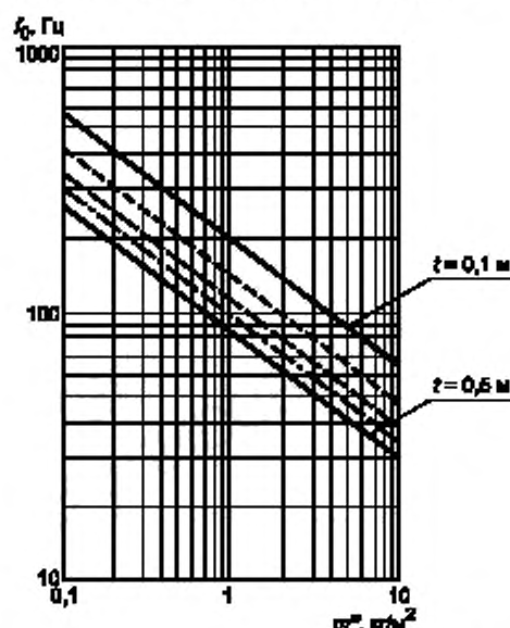
Рисунок 15 — Зависимость резонансной частоты f_0 пластиначного или пленочного резонатора от поверхностной плотности массы m'' податливой пластины перед разделенной на секции облицовкой глубиной t ( c = 340 \text{ м/с} , \rho = 1,2 \text{ кг/м}^3 )
