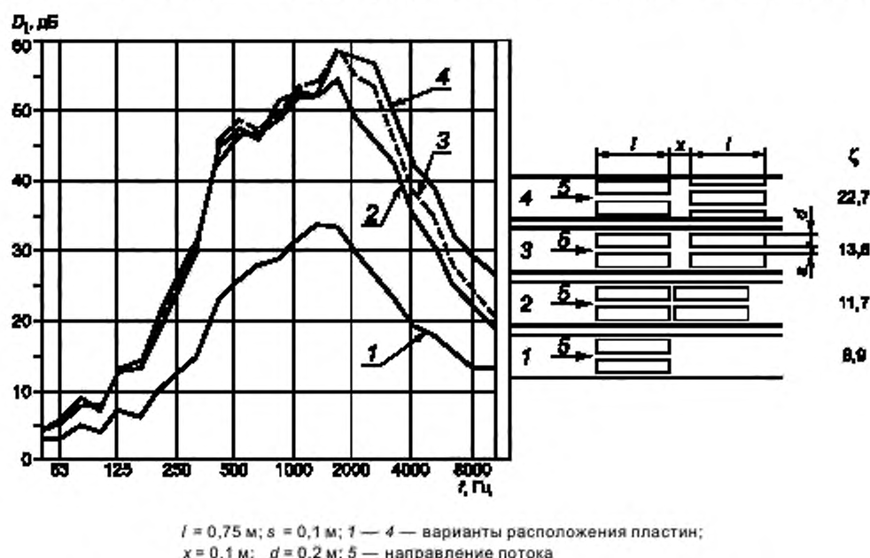
Рисунок 9 — Экспериментально полученные зависимости вносимых потерь D_1 от частоты f и коэффициента потери давления \zeta для различных вариантов расположения пластин
