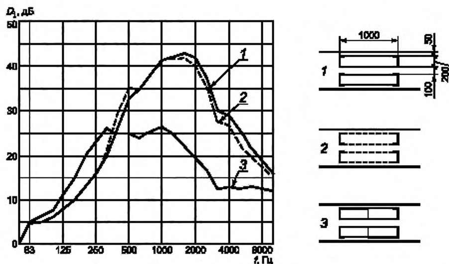
Рисунок 7 — Зависимость удельных потерь распространения D_n от частоты f для глушителя с пластинами разной толщины и ширины воздухопроводов между пластинами, равной толщине пластин
