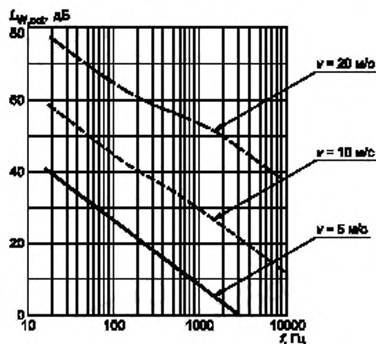
Рисунок 10 — Зависимость октавных уровней звуковой мощности L_{W_{окт}} потокового шума от частоты f при нормальных атмосферных условиях для канального глушителя с площадью наименьшего поперечного сечения S = 0,5 м 2 , максимальным поперечным сечением канала H = 1 м при различных скоростях потока v
