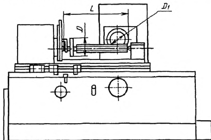
D — наибольший диаметр устанавливаемого изделия; L — наибольшая длина устанавливаемого изделия; D_1 — наибольший диаметр шлифовального круга
