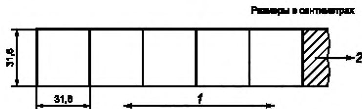
Рисунок 1 — Метод отбора образцов для матов
