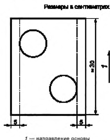
Рисунок 3 — Предлагаемый метод вырезания образцов ткани шириной от 25 до 50 см
