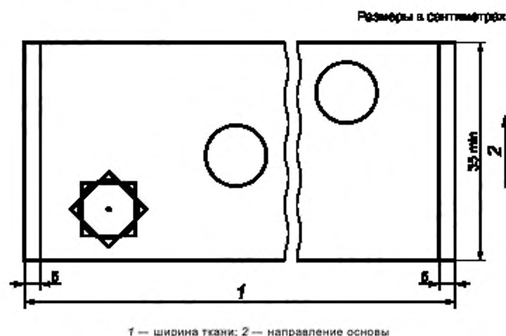
Рисунок 2 — Предлагаемый метод вырезания образцов ткани шириной больше 50 см
